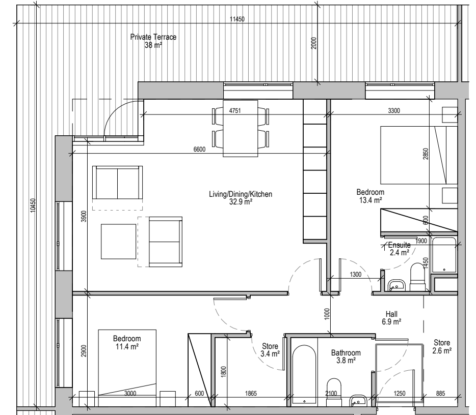
③ AT02a 2 BED 78 SQM 1 : 100
