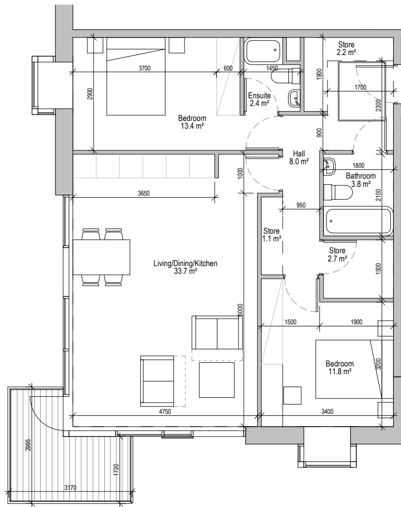
① AT01 2BED 82.3 SQM 1 : 100
